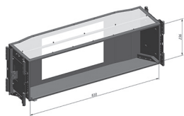
Die Aufzugsklappe
